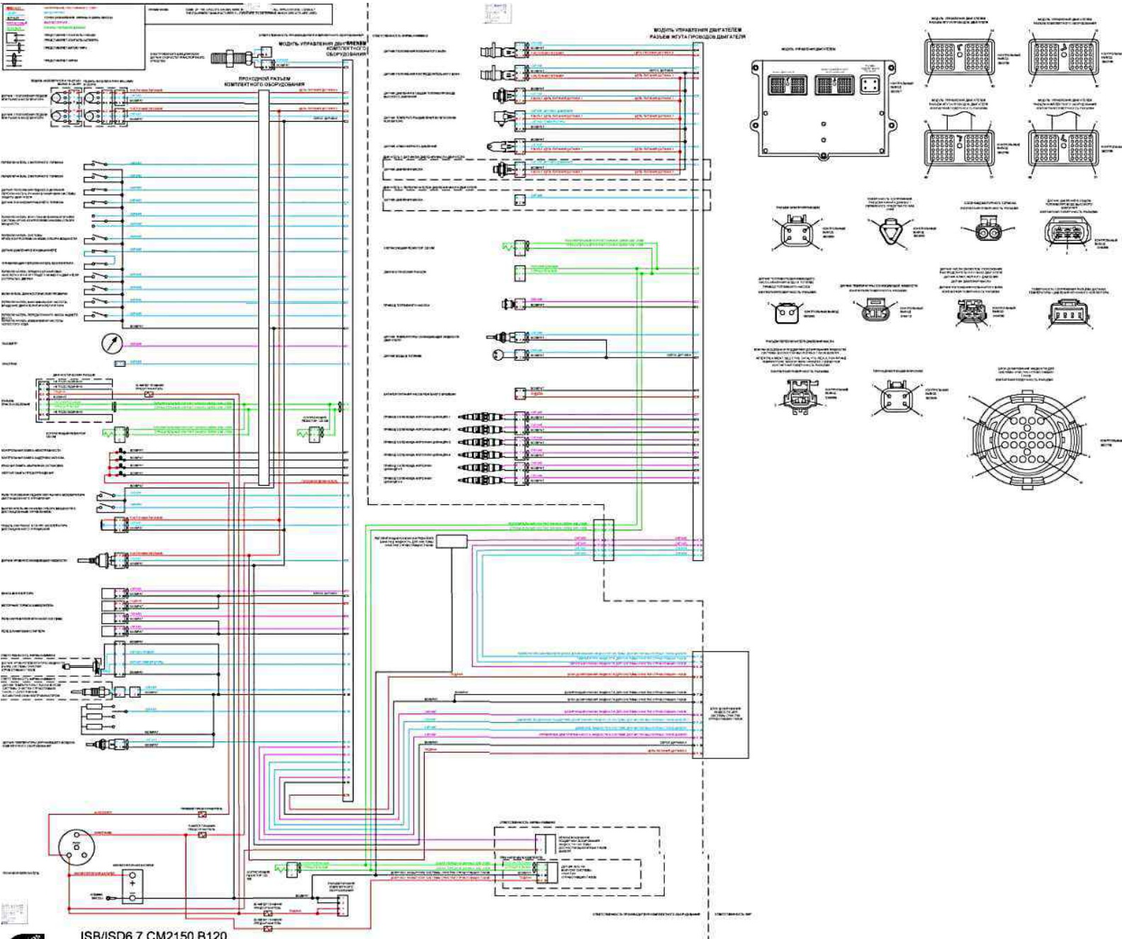
ISB/ISD6.7 CM2150 B120 СХЕМА ЭЛЕКТРИЧЕСКИХ СОЕДИНЕНИЙ БЕЛЫЙ ОБЪЕКТ ОТДЕЛЕНИЕ В СВА 15 МАРТ 2014
