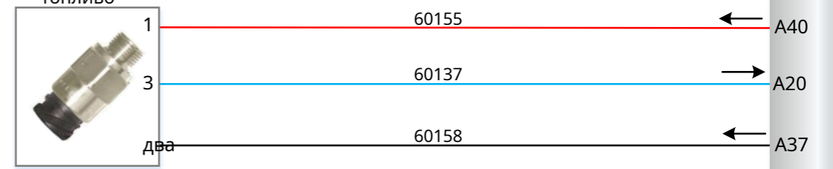
датчик давления ТОПЛИВО
