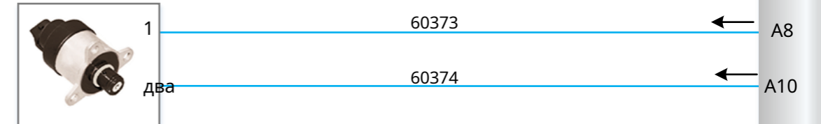
пропорциональный клапан ТОПЛИВО
