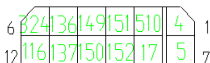
C016;12针脚 仪表线束-顶棚线束
