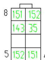
C109, 8针脚 仪表线束-遮阳帘左
