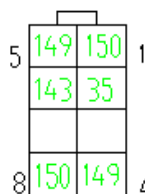
C108, 8针脚 仪表线束-遮阳帘开 关右
