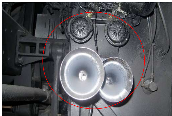
Позиция гудка: Находится под сидением водителя назади усилителя руля
